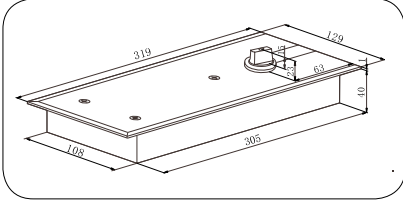
20-112 Üst Düz Menteşe/Upper Hinge
