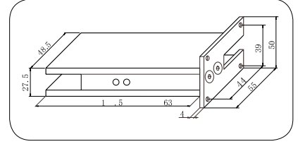
20-122 Karşılık/Lock Strike
