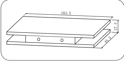
20-119 Üst Menteşe Karşılığı/Bearing Base
