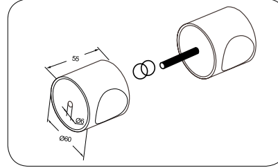
20-132 Cam Kapı Kolu/Metal Handle
