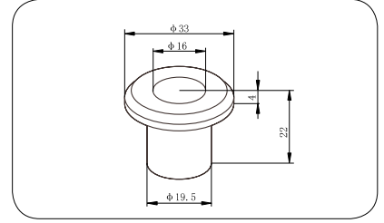
21-132 Cam Kapı Kolu/Metal Handle
