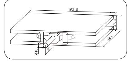
20-114 T Menteşe/T Hinge
