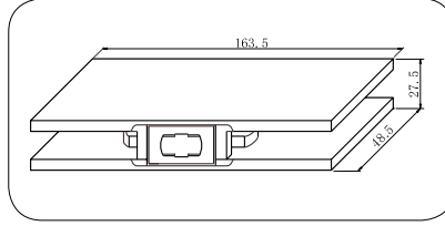
20-113 Küçük Menteşe/Small Single Hinge
